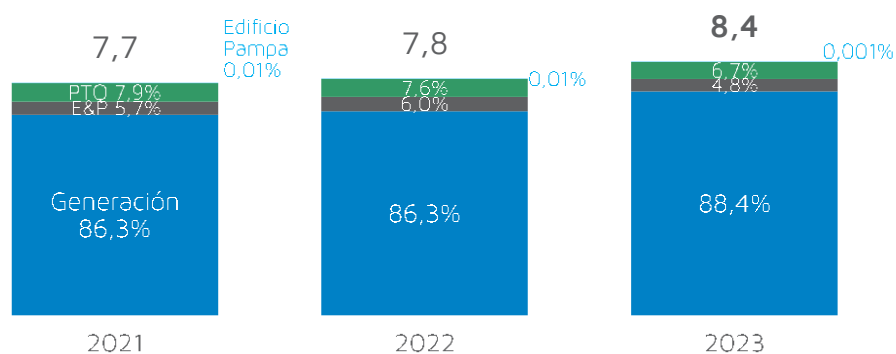
Evolución de las emisiones Por negocio, en millones de tCO 2 e
